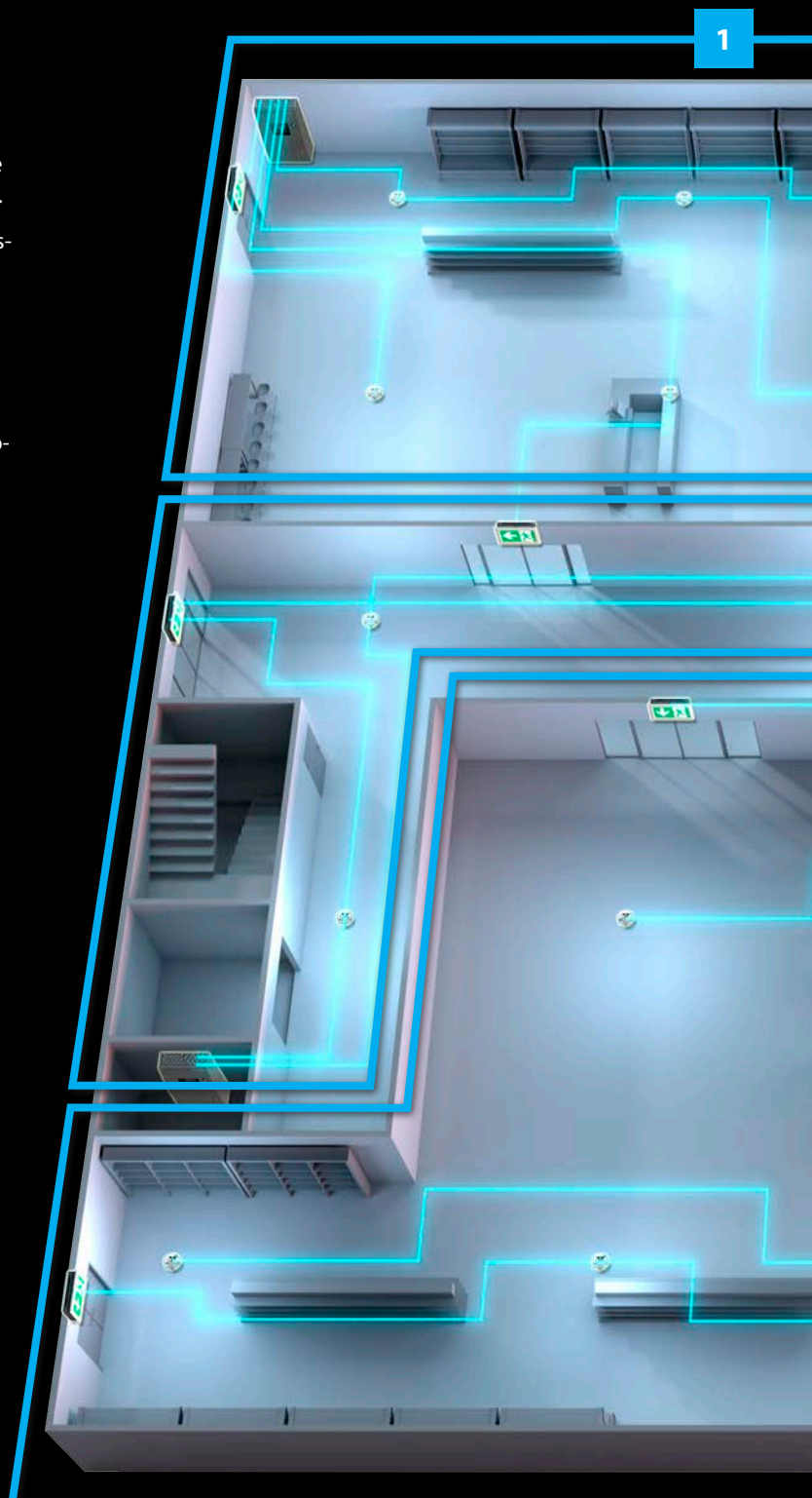
Brand-/Sicherheitsbeleuchtungsabschnitte
